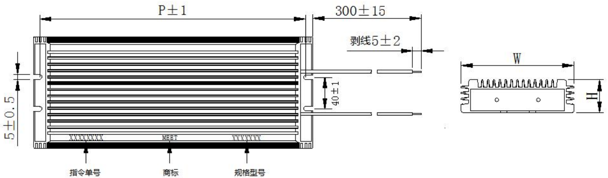
图二(俯视图)
